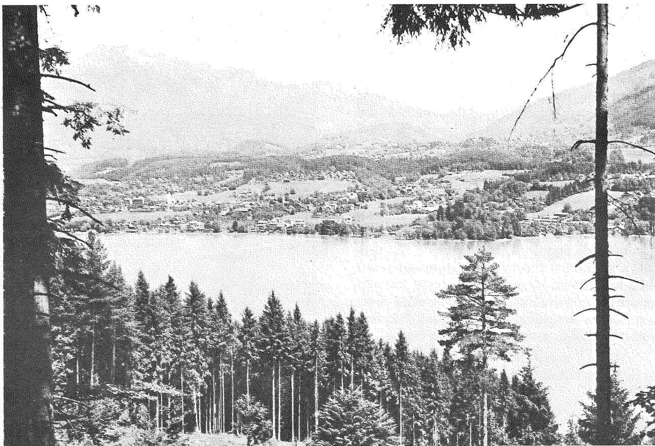
Näkymä Seebodenista.
